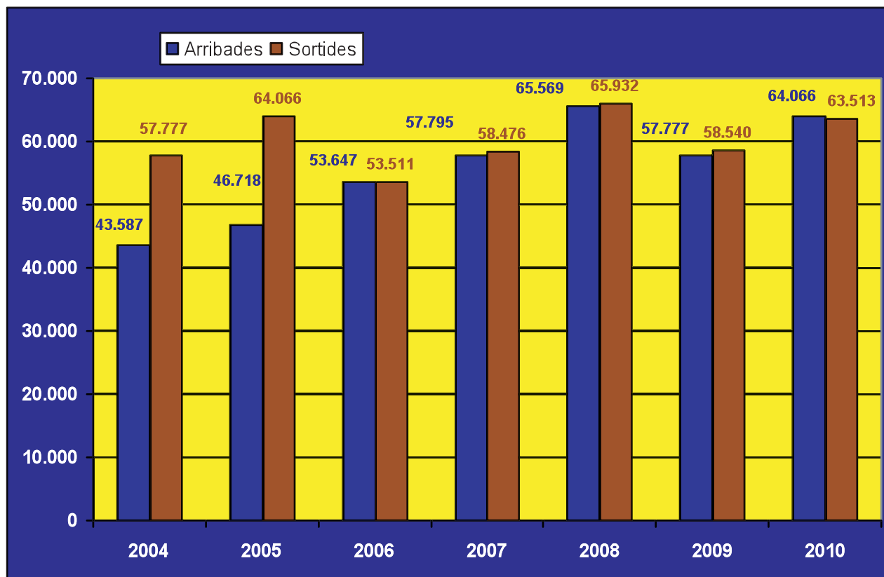
Figura 6.1: Arribades i sortides amb AVE a Lleida en el primer trimestre de cada any (2004-2010)
