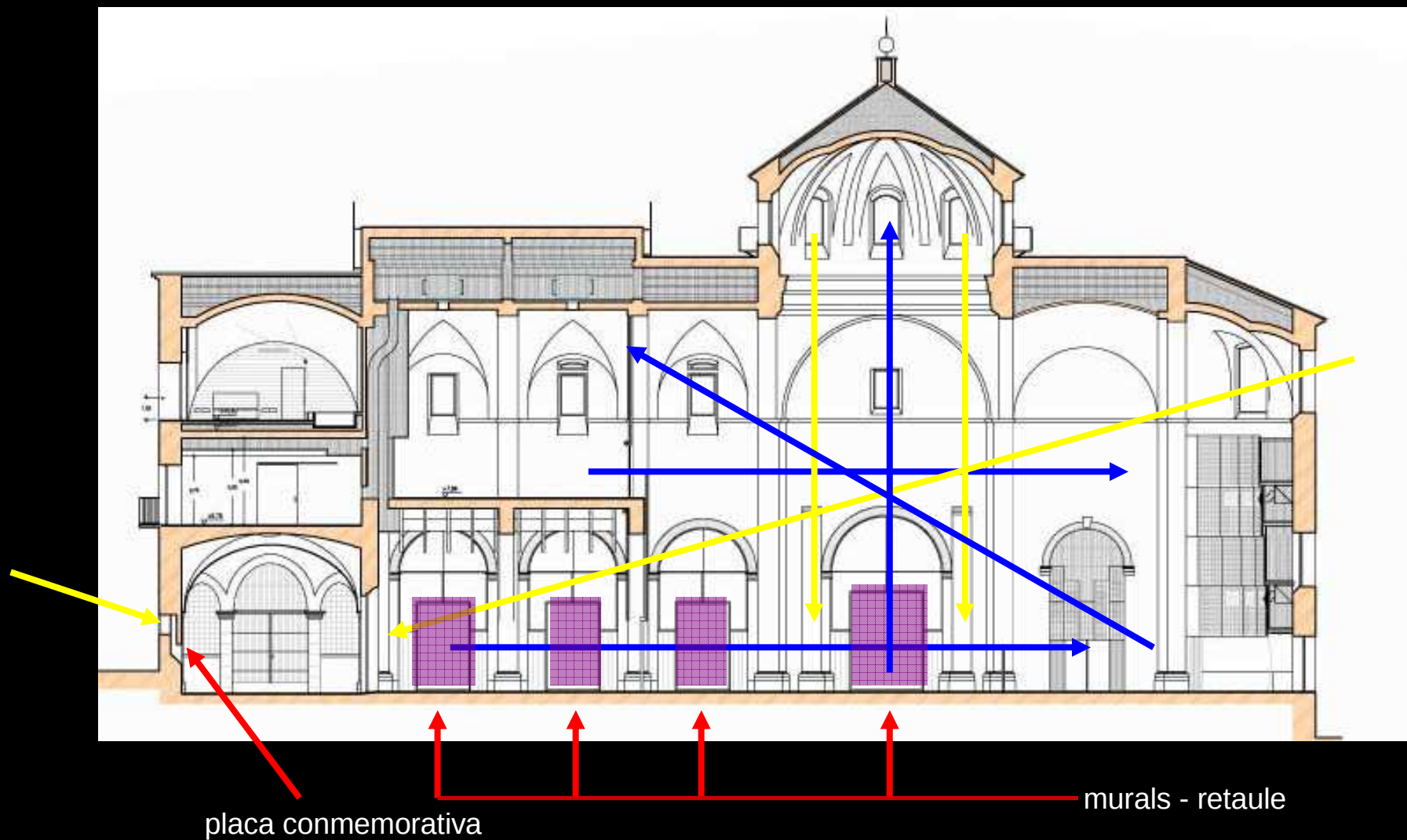
Secció longitudinal església
