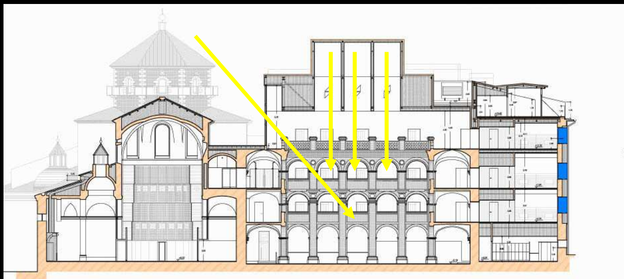
Seccions llevant - ponent
