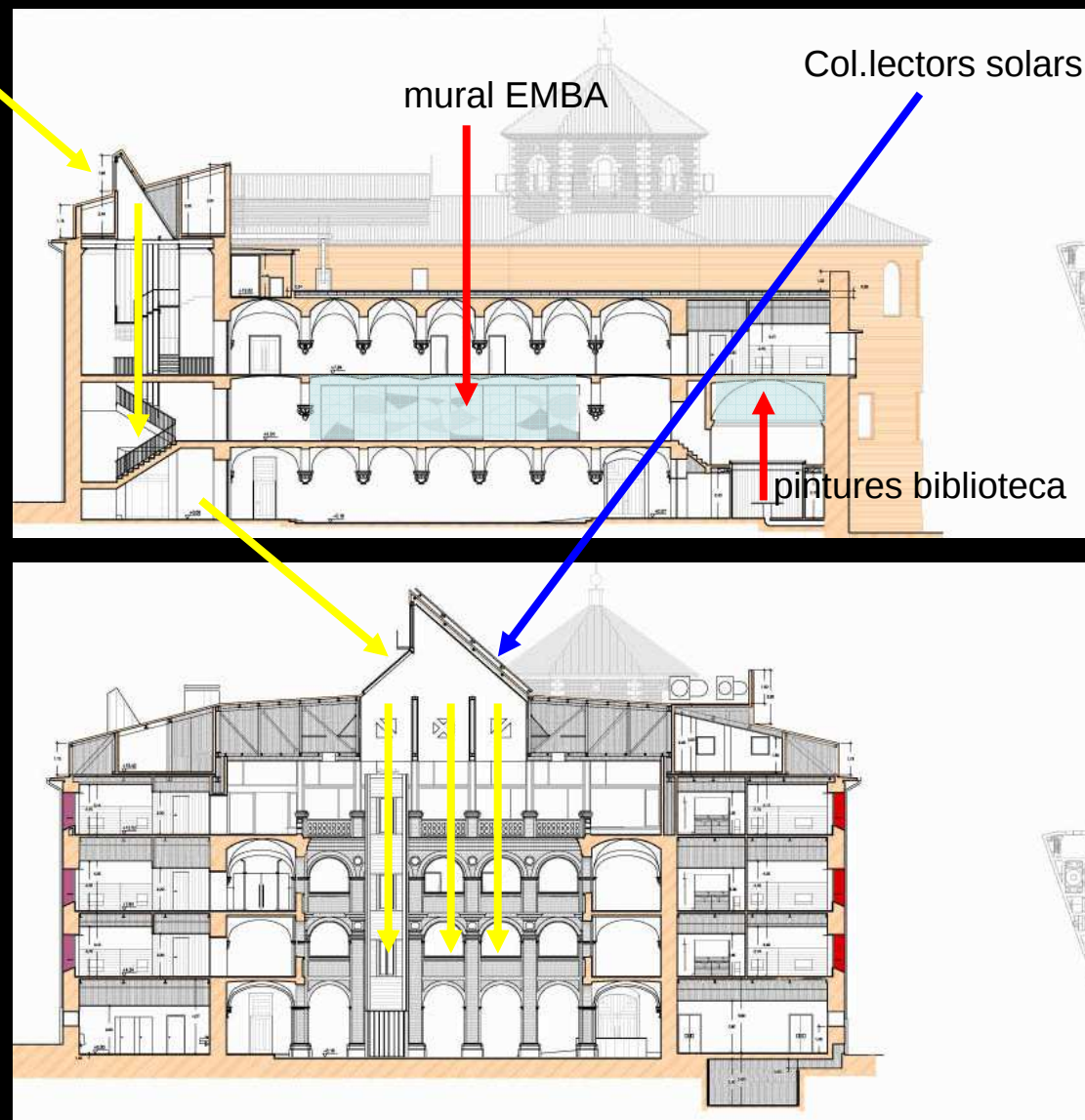
Seccions nord - sud
